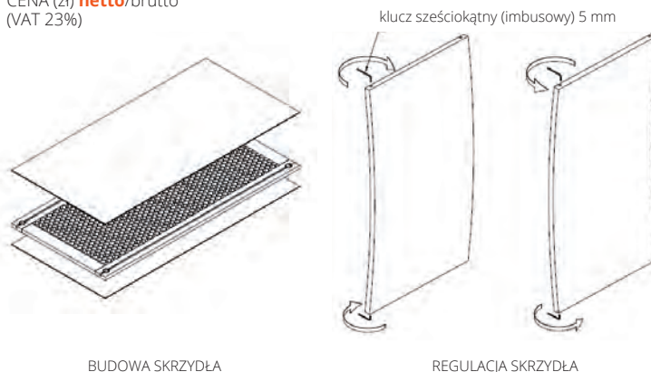
BUDOWA SKRZYDŁA
