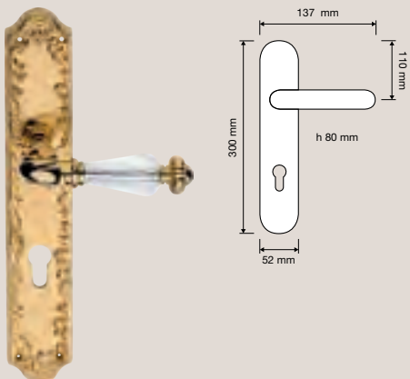
1543 PL Maniglia con placca art.1397 / Door handle on plate art.1397
