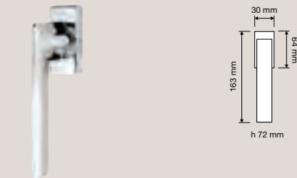
1425 DK Maniglia per finestra con movimento DK 4 posizioni / Window handle with DK movement 4 clicks
