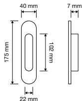
Chic 1670 IP Placca incasso su placca / Flush pull on plate
