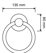
Leone 351 BA 110 Battente con anello / Door knocker with ring
