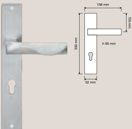
1410 PL Maniglia con placca / Door handle on plate
