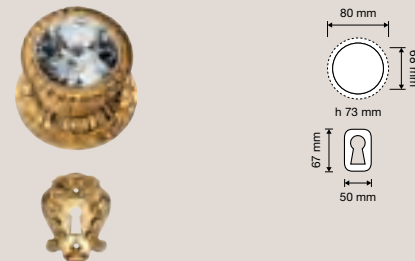
1545 PG Pomolo a girare con rosone art.1540 / Turnable knob on big rose art.1540
