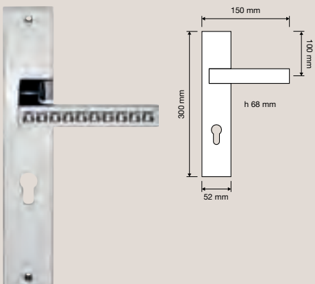
1216 PL Maniglia con placca art.1104 / Door handle on plate art.1104
