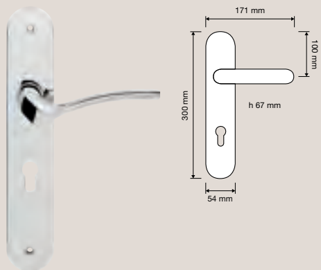
719 PL Maniglia con placca art.1595 / Door handle on plate art.1595
