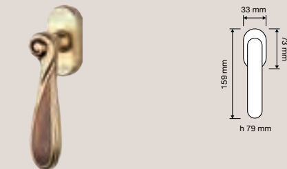
1650 SK Maniglia per finestra con movimento DK SmartBlock / Window handle with DK SmartBlock movement
