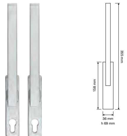
Zen 1615 MC Maniglione alzante accoppiato foro yale / Set pull handles cylinder hole
