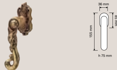
1395 DK Maniglia per finestra con movimento DK 4 posizioni / Window handle with DK movement 4 clicks
