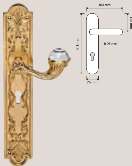
1530 PL Maniglia con placca art.1405 / Door handle on plate art.1405
