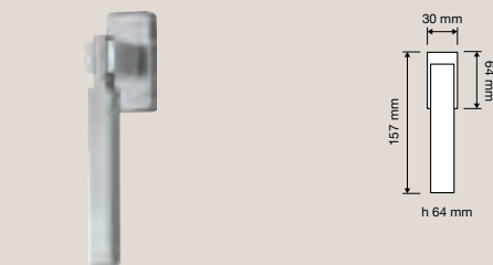
1050 DK Maniglia per finestra con movimento DK 4 posizioni / Window handle with DK movement 4 clicks
