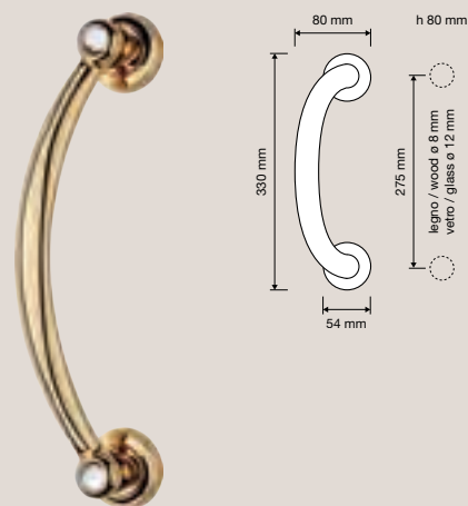
991 MN 275 108 Maniglia con rosette art.108 / Pull handle on roses art.108
