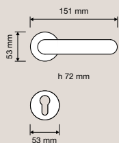
1563 IP Placca incasso su placca Small / Flush pull on plate Small
