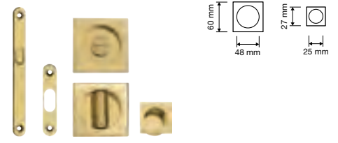
184 KT Kit incasso quadrato con nottolino, taglio cacciavite, maniglia trascinamento e serratura / Square inset handle kit with thumb, finger pull and locking system
