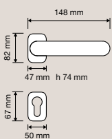
1535 DK Maniglia per finestra con movimento DK 4 posizioni / Window handle with DK movement 4 clicks
