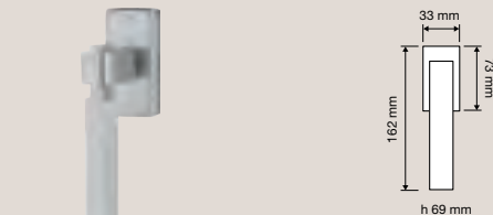
1050 SK Maniglia per finestra con movimento DK SmartBlock / Window handle with DK SmartBlock movement
