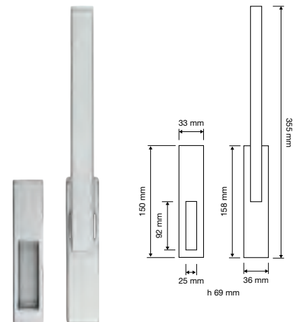
Zen 1615 MN Maniglione alzante singolo con nicchia / Single pull handle with flush pull
