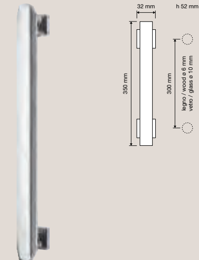
1555 MN 300 Maniglione. Interassi disponibili 300-400- 600. / Pull handle. Available distances 300-400-600.
