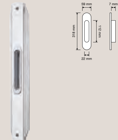
1555 IP Placca incasso su placca / Flush pull on plate
