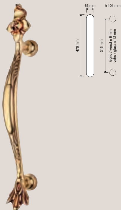
1408 MN 723 Maniglione Crystal. Attenzione: l'interasse può variare leggermente, chiedere sempre le misure prima di forare la porta. / Crystal pull handle. Attention: the distance can have little changes, please always ask before making the holes in the door.
