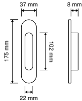
Beta 488 IP Placca incasso su placca / Flush pull on plate
