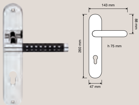
1726 PL Maniglia con placca art.123 / Door handle on plate art.123
