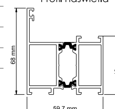
Profil naświetla
