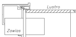
wariant 1 otwierany na zewnątrz ODZ lustro od strony przeciwnej do zawiasów (A/Z)
