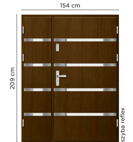
NS 33 Widok od zewnątrz Dostawka stała - imitacja skrzydła
