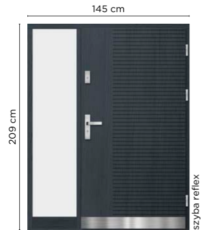
NS 22 Widok od zewnątrz Dostawka stała w ościeżnicy
