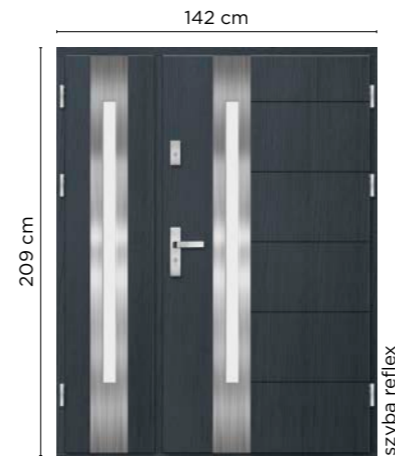
NS 23 Widok od zewnątrz Dostawka stała - imitacja skrzydła
