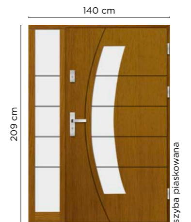
NS 37 Widok od zewnątrz Dostawka stała w ościeżnicy
