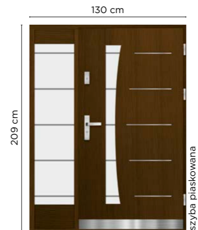
NS 34 Widok od zewnątrz Dostawka stała w ościeżnicy
