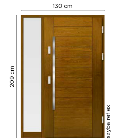
NS 36 Widok od zewnątrz Dostawka stała w ościeżnicy
