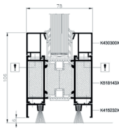
przekrój dolny drzwi bez progów
