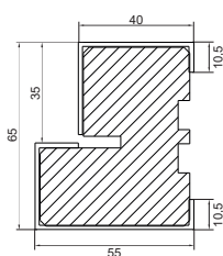
Ościeżnica drewniano-stalowa DS/54
