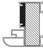
Drewniano-aluminiowa PASSIVE/90
