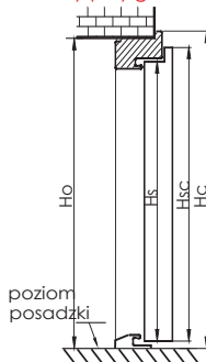
Drzwi trzy przylgowe 3P
