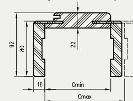
Przekrój poziomy OR/ORC
