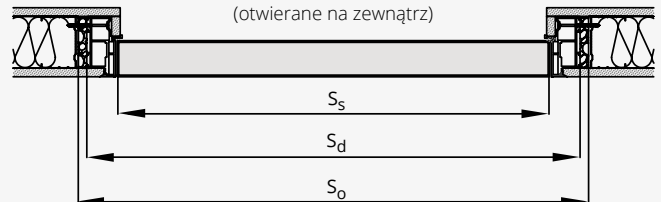
DRZWI OTWIERANE NA ZEWNĄTRZ ODZ
