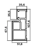
Rysunek techniczny
