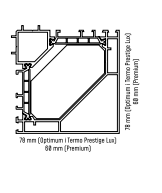
Rysunek techniczny
