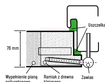
PROFIL SKRZYDŁA
