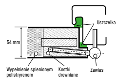
PROFIL SKRZYDŁA
