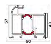
Rysunek techniczny
