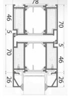
Rysunek techniczny
