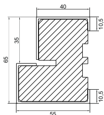
Ościeznica drewniano-stalowa DS/54
