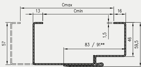
Profil ościeżnicy OSR z kątownikiem domykającym T57
