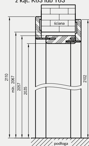
Przekrój pionowy tunelu regulowanego z ką. K63 lub T63
