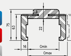
Przekrój OR/ORC z ką. K63
