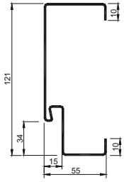
Ościeznica stalowa S15/54
