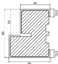
Ościeznica drewniano-stalowa DS/54
