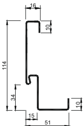
Ościeznica stalowa 11/54, 11/54 AKU
