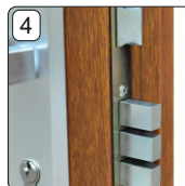
4 Zamek podstawowy klasy 4
