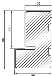
Ościeżnica drewniano-stalowa DS/75
