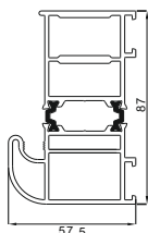
Ościeżnica aluminiowa ALU/75
