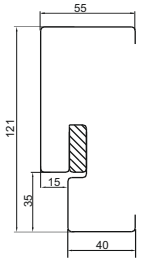
Ościeznica stalowa T/54, T/54 AKU
