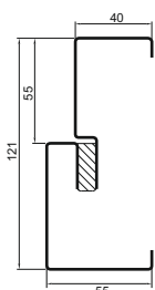
Ościeżnica stalowa NT/75
