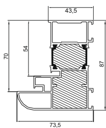
Ościeżnica aluminiowa ALU/90
