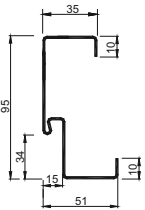
Ościeznica stalowa 10/54, 10/54 AKU
