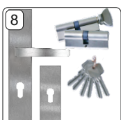
8 Klamka SIGMA, wkładka+wkładko-gałka system jednego klucza standard
