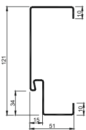
Ościeznica stalowa 15/54, 15/54 AKU
