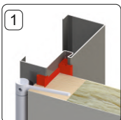
1 Wypełnienie skrzydła PŁYTA SKALNEJ WEŁNY MINERALNEJ
