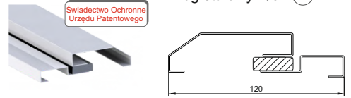
Próg stalowy T/54 (3P)
