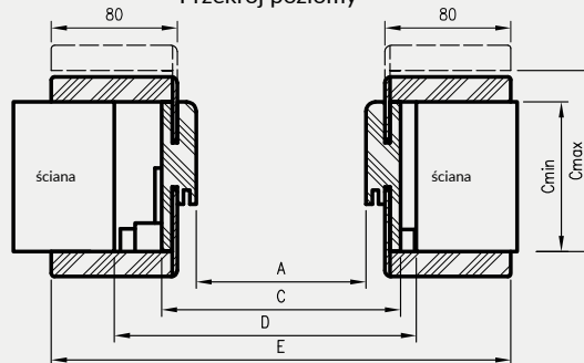
D - wymagana szerokość otworu w murze
