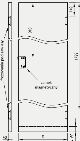
Skrzydła Sara Eco bezprzylgowe
