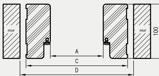
Przekrój poziomy OP
