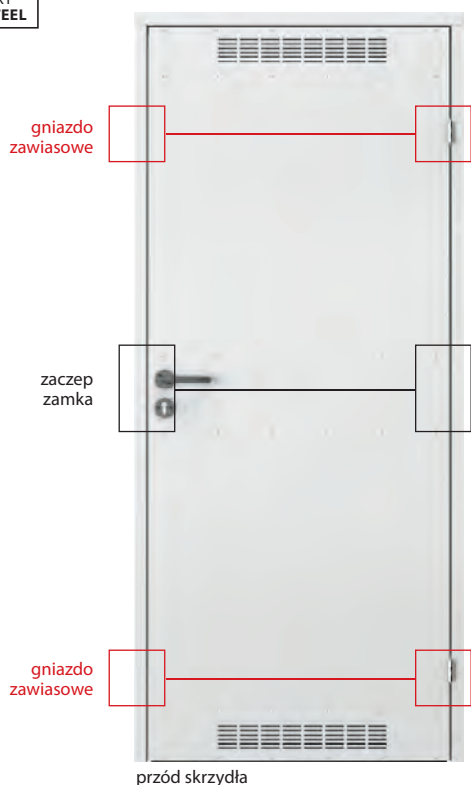
przód skrzydła
