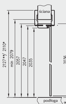
Przekrój pionowy drzwi szklanych z ORC
