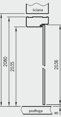
Przekrój pionowy drzwi szklanych
