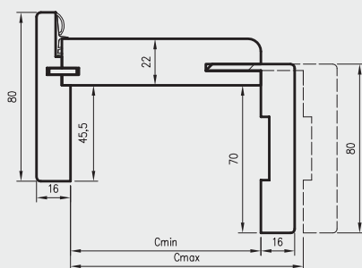
Przekrój pionowy ORO
