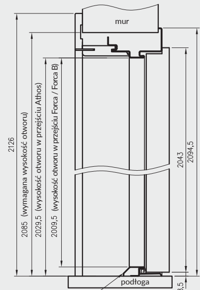
przekrój pionowy
