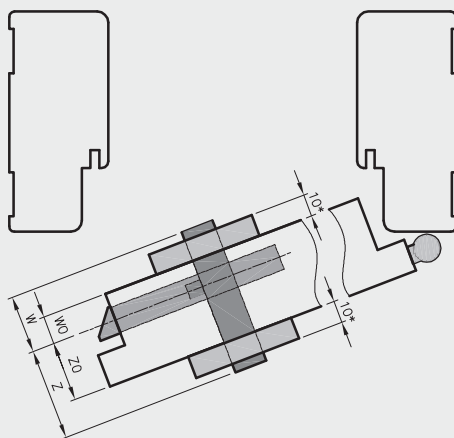
Rys. Dobór wymiaru wkładki bębnekowej
