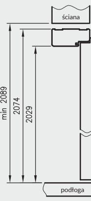
Przekrój pionowy drzwi przylgowych
