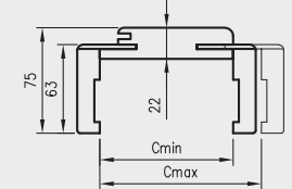
Przekrój OR/ORC z ką. T63
