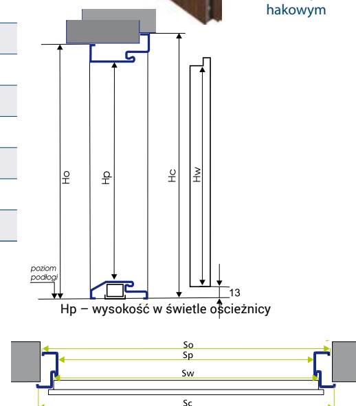
drzwi z zamkiem listwowym hakowym
