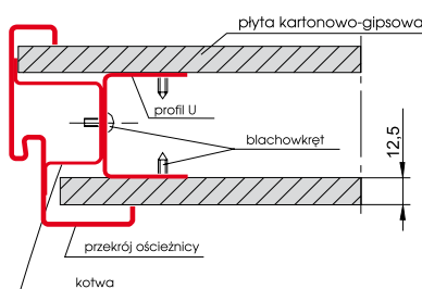
Osadzanie w ścianie kartonowo-gipsowej
