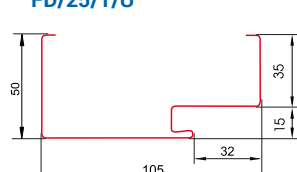
FD/25/1/U
