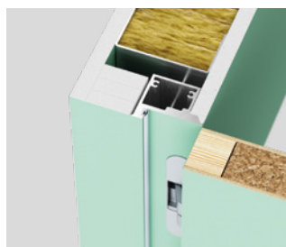
Bezprzylgowe standard (otwierane na zewnątrz) - drzwi prawe
